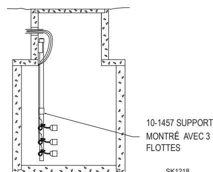
SUPPORT DE FLOTES TYPIQUE POUR PUISARD EN BÉTON OU POUR PUITS D'ACCÈS DE FOSSE SEPTIQUE
