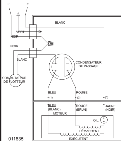
SCHÉMA ÉLECTRIQUE POUR LES MODÈLES
